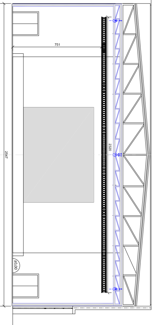
Salle de la Manufacture - CREIL Vue fond de Salle - Elevation Juin 2009 Echelle 1/200 Dimensions en cm
